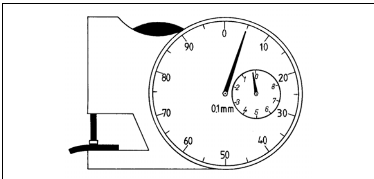
Abb. 4.1-4: Handdickenmesser
